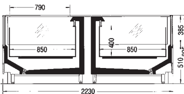
Ivando SG4.B4/B8
