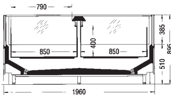
Irios SG4.B4/B8
