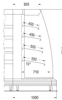
Marena 73.CE A4
