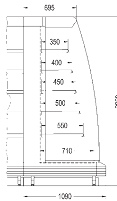
Marena 73.CE A3 L
