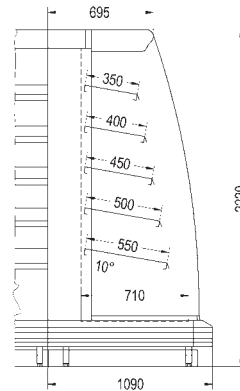
Marena 73.CE A4 L
