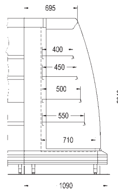
Marena 73.CE A3
